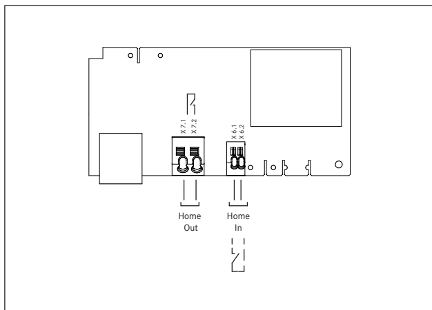
Fig. 6.31 Koblingsskjema for eksterne bryterkontakter
