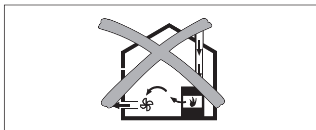
Fig. 6.23 Uttrekkingsmontering – ikke tillatt
