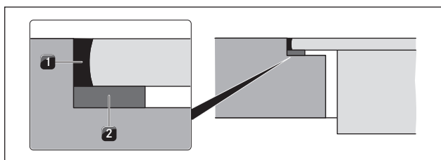
Fig. 6.6 Tetningsbånd ved planlimt montering
