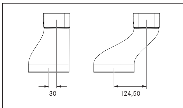
Fig. 6.10 Forskyvning med overgangsstykker
