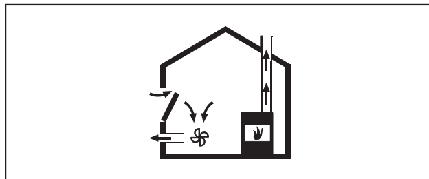
Fig. 6.24 Uttrekkingsmontering – korrekt
