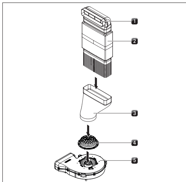
Fig. 6.17 Montering
