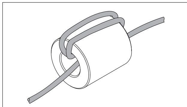
Fig. 6.29 Vikle tilkoblingsledningen 3 ganger rundt ferritthylsen
