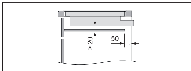
Fig. 6.8 Sidevisning kabelbeskyttelsesgulv og ventilasjon
