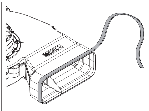
Fig. 6.20 Posisjon tetningsbånd for montering med overgangsstykke (flatkanal)
