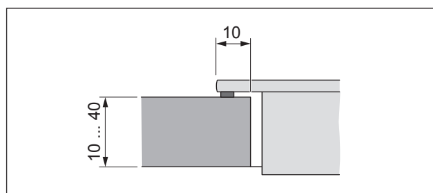
Fig. 6.5 Snitt overflatemontering
