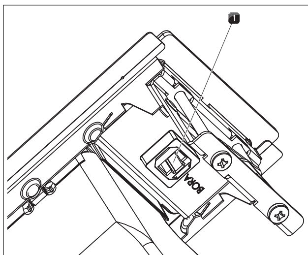
Fig. 6.26 Tilkobling kommunikasjonsledning CAT 5
