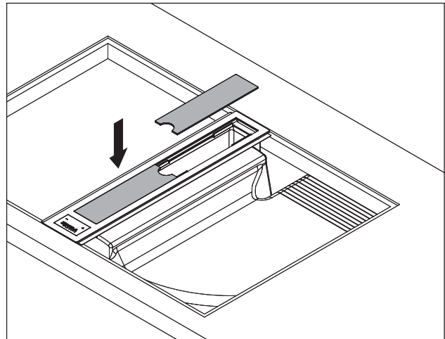
Fig. 8.4 Sette inn dekkeplatene
