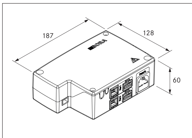
Fig. 6.11 Monteringsmål Universal styringsenhet
