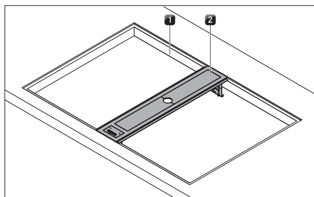
Fig. 6.13 Montere avtrekk
