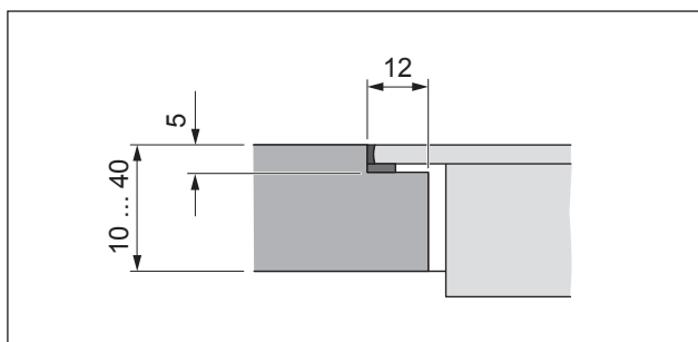
Fig. 6.3 Snitt falsemål
