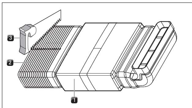
Fig. 6.16 Forkorte Silence-modul
