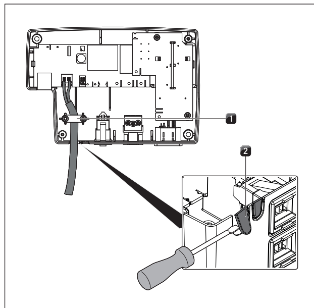
Fig. 6.32 Kontakt Home-Out med strekkavlastning
