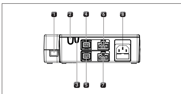
Fig. 6.25 Tilkoblinger for Universal styringsenhet USEE
