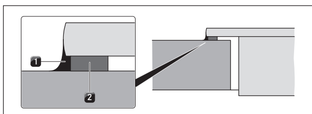
Fig. 6.7 Tetningsbånd ved overflatemontering
