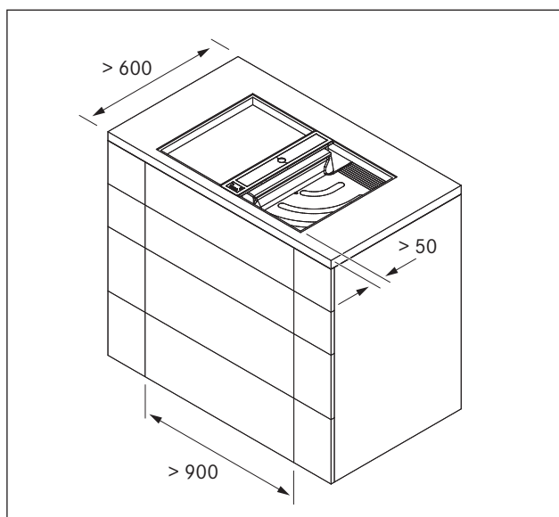
Fig. 6.12 Apparatmonteringsmål
