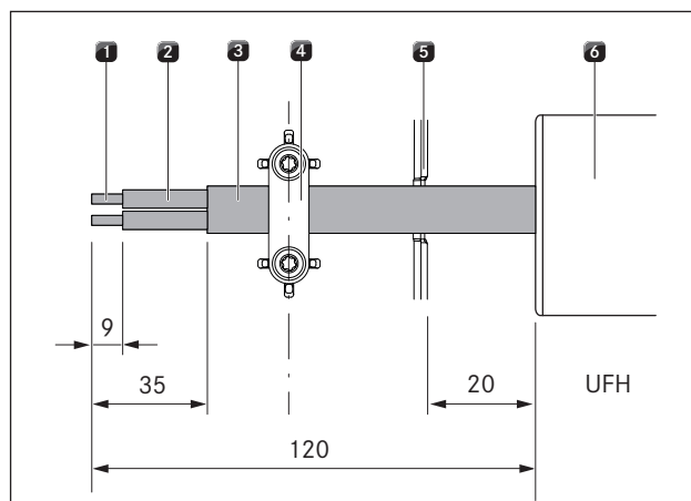
Fig. 6.30 Avisoleringslengder og monteringsposisjon for tilkoblingsledningen i Universal styringsenhet
