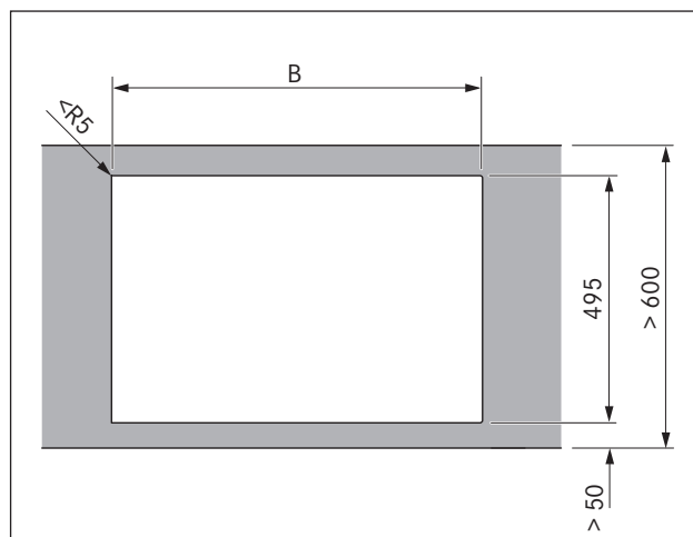
Fig. 6.4 Overflatemontering
