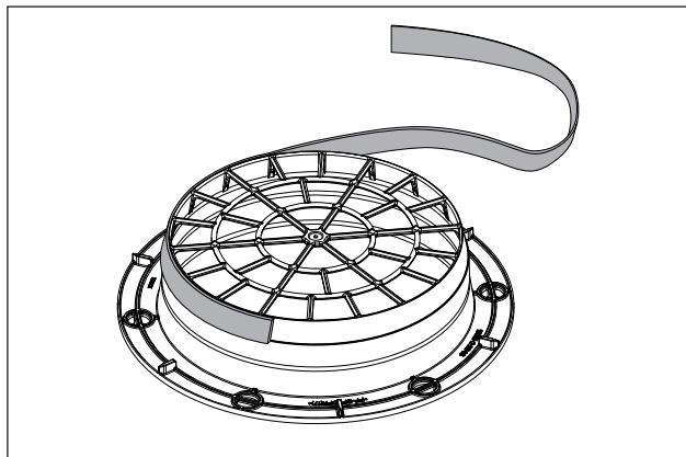
Fig. 6.19 Posisjon tetningsbånd for montering med rundrør
