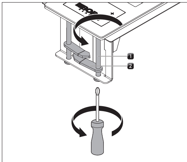
Fig. 6.15 Feste avtrekket
