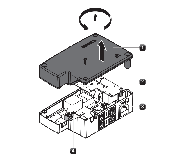
Fig. 6.28 Åpne deksel til Universal styringsenhet
