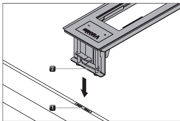
Fig. 6.14 Høydejusteringsplater
